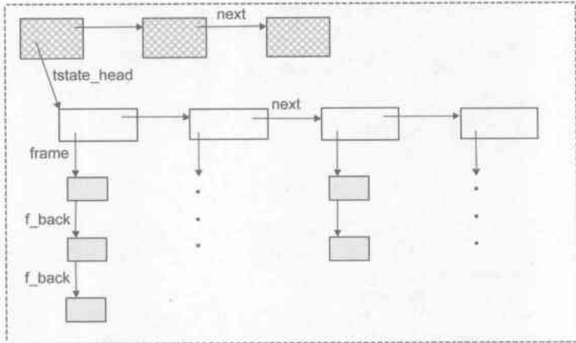
图 8-6 Python 的运行时环境
